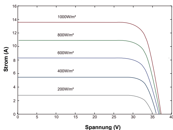
Strom-Spannungs Kurve (TT405-108PM10)
